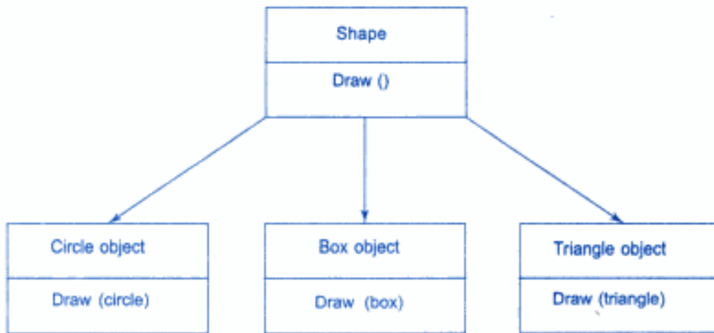
Fig. 1.9 ⇔ Polymorphism
